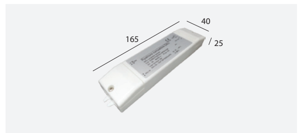
Opto-isolator 48V DALI
